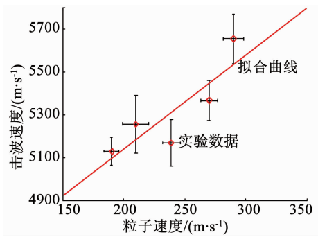
图 5 材料的 D - u 曲线
