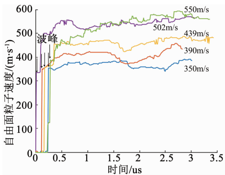
图 4 自由面速度
