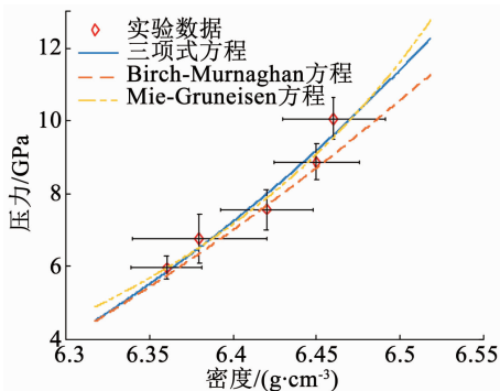
图 8 材料物态方程曲线
